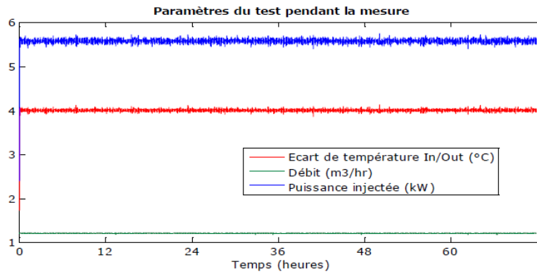
Figure 3 : Exemple d'évolution de différence de température ( T_e-T_s ), de débit et de puissance échangée pendant un TRT. Source : Rapport BRGM/RP-60816-FR
